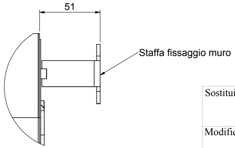
DETTAGLIO Y SCALA 1 : 2
